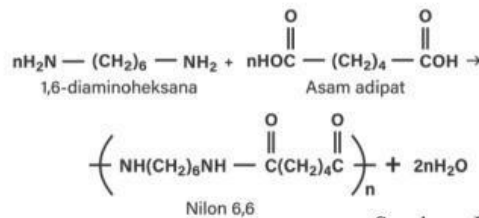
Gambar 2. 2 Pembentukan nylon-66
