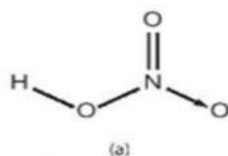
Cấu tạo phân tử nitric acid (a), mô hình phân tử nitric acid (b), nitric acid được bảo quản trong lọ thủy tinh tối màu (c)
