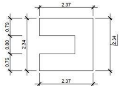
PLANTA ESCALA 1:75
