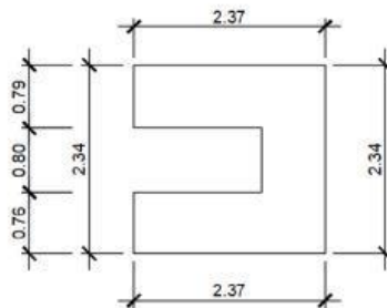
PLANTA ESCALA 1:75
