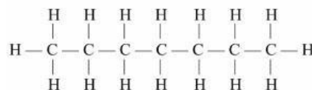
Struktur n-heptana
