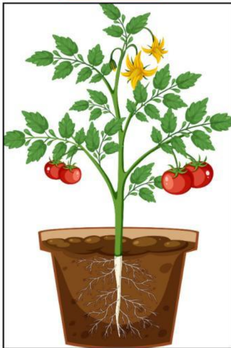
Tumbuhan 1
