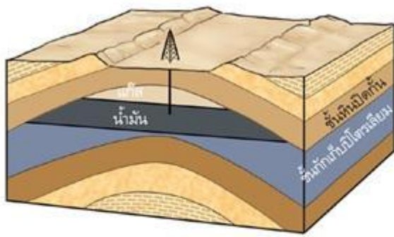
กักเก็บในโครงสร้างแบบประทุนคว่ำ
