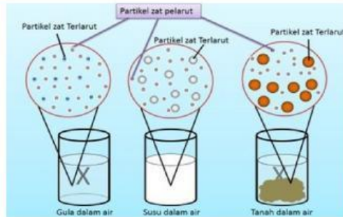
Gambar 3. Perbedaan partikel zat terlarut
