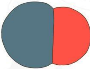
Gambar 11. Satu Molekul Karbon Monoksida (CO) (Canva, diakses 2025)
