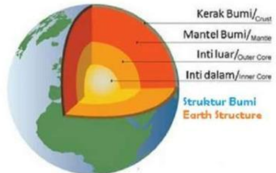
Gambar 2 Struktur lapisan bumi Sumber: Google.com
