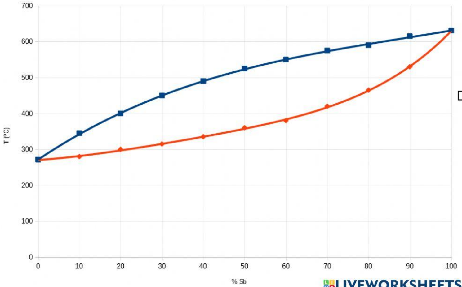
Diagrama Sb - Bi
