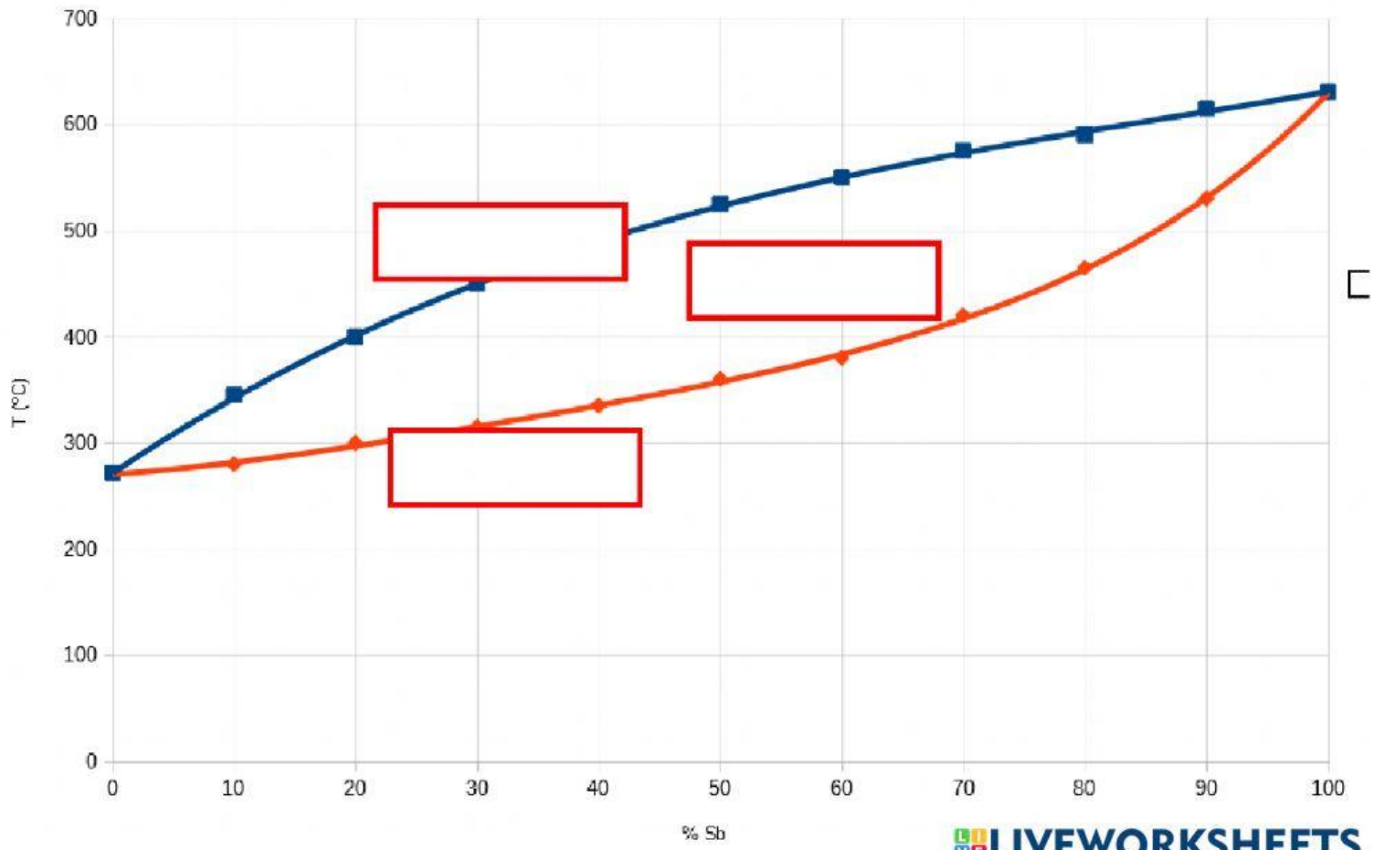
Diagrama Sb - Bi
