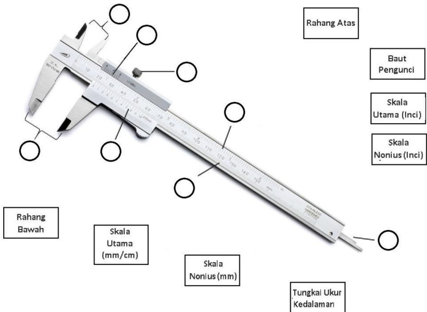
Bagian-Bagian Jangka Sorong
