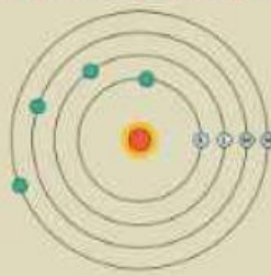
Gambar 7. Atom Bohr
