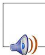
_ ff _ n
