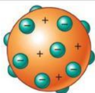
MODELO DE THOMSON
