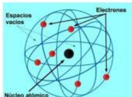
MODELO DE RUTHERFORD
