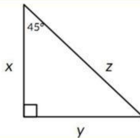
Gambar 4.12 Segitiga dengan Sisi XYZ
