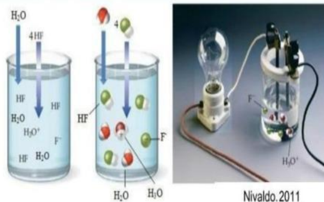
Gambar 22. Ionisasi larutan HF dan daya hantar listrik larutan HF
