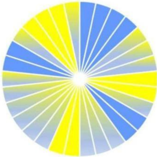
Діаграма хмарності за січень 2024 р.
