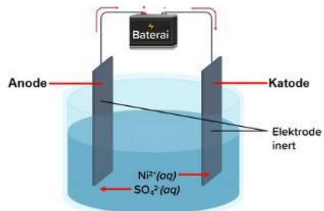
Sel Elektrolisis
