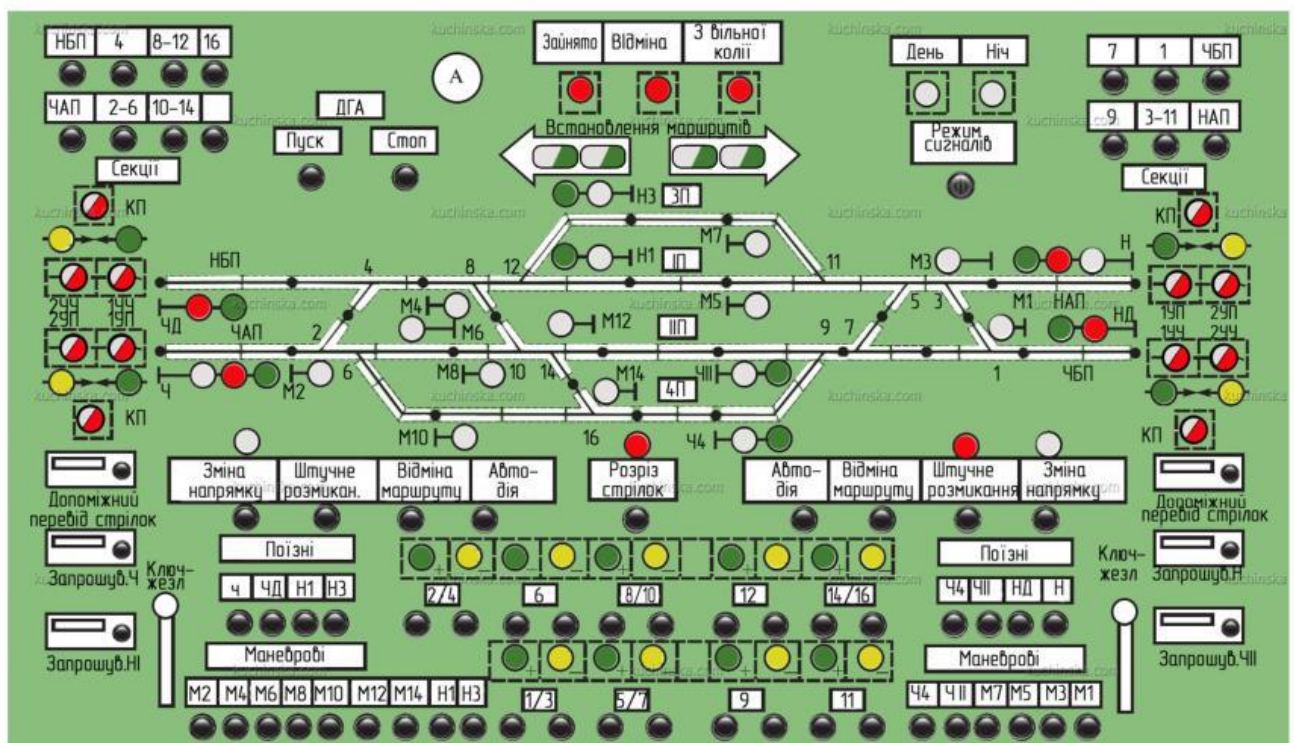
Рис. 9.1 - Пульт управління уніфікованого типу
