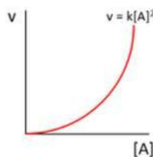
Gambar 3. Grafik reaksi orde 2
