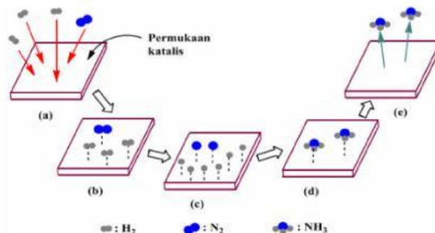
Gambar: Reaksi antara molekul-molekul \text{N}_2 dan \text{H}_2 membentuk molekul \text{NH}_3 pada permukaan katalis \text{Fe} .
