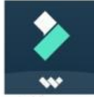
Filmora
