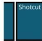
Shotcut
