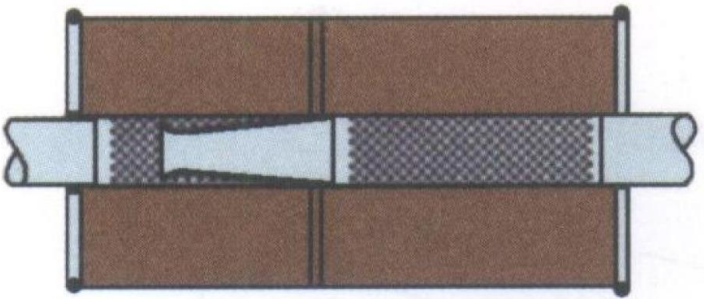
a) absorbční tlmič výfuku
