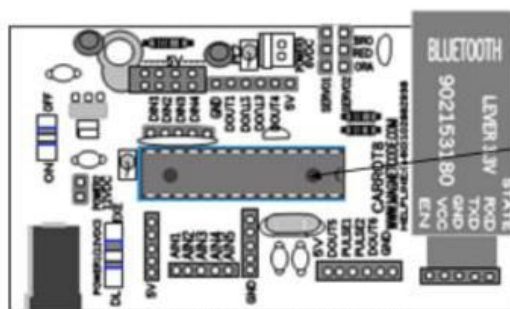
Papan litar elektronik mikropengawal
