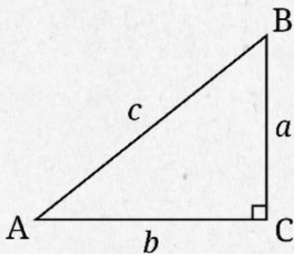
Gambar 1.4 Segitiga Siku-siku
