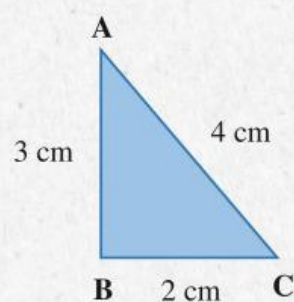
Gambar 1.5 Segitiga Sebangun
