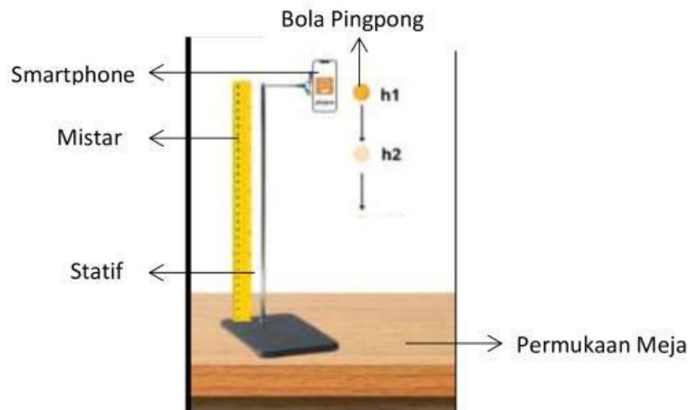
Gambar 1. Skema Praktikum Koefisien Restitusi dan Persentase energi yang hilang
