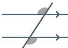
Sudut luar bersebrangan
