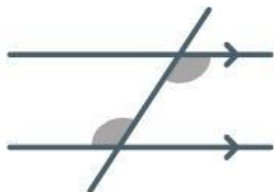
Sudut dalam bersebrangan
