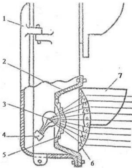
Рисунок 2.1 - Лінзовий комплект
