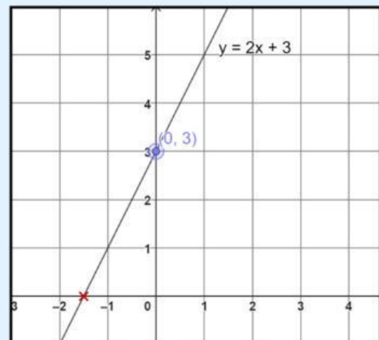
Gambar 1.3 Garis lurus dari persamaan y = 2x + 3
