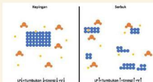
Gambar 3. Tumbukan Partikel
