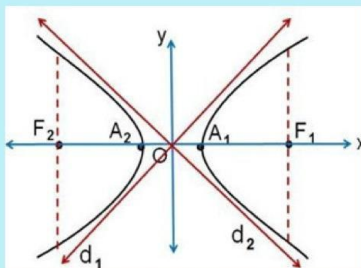
Hiperbola horizontal
