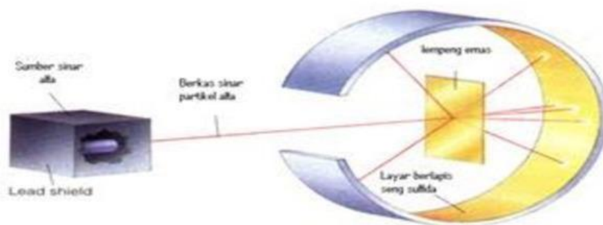
Gambar 6: Eksperimen Rutherford
