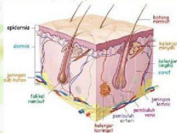
Gambar 3. Struktur kulit
