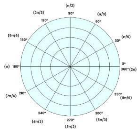
Graph B(-2, 150^\circ)
