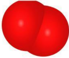
Molekul O 2
