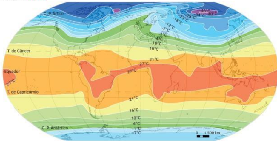
Fig. 2 Distribuição das temperaturas médias (°C) de janeiro, reduzidas ao nível do mar.
