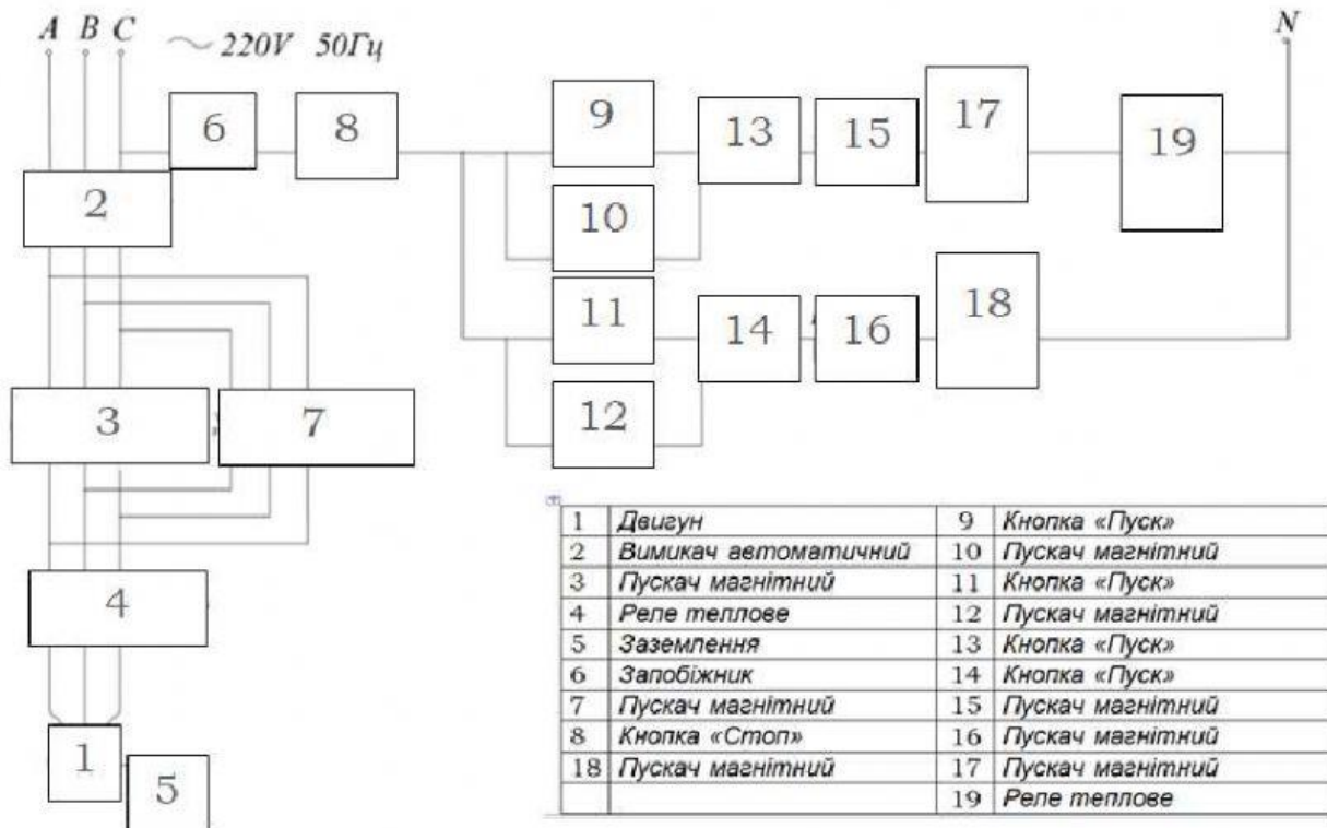
Схема реверсивного пуску асинхронного двигуна з КЗ ротором
