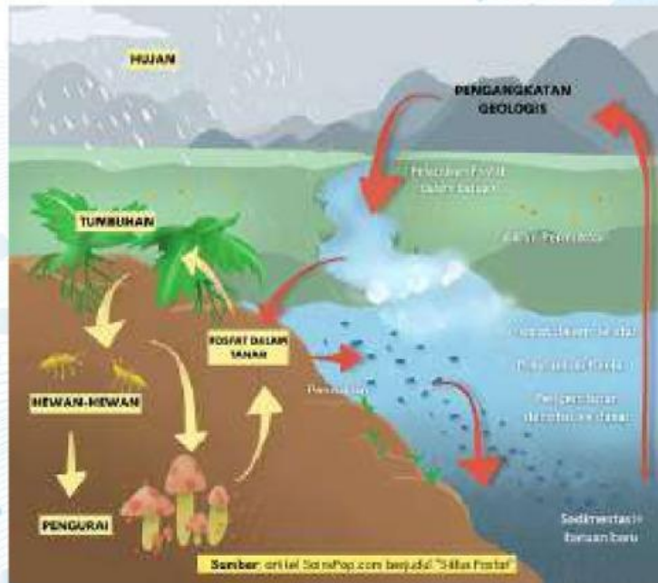
Siklus Fosfor
