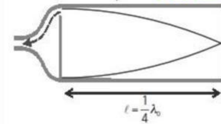
Gambar 2. 10 . Pipa Organa Tertutup Nada Dasar
