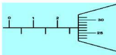
Soal mikrometer sekrup nomor 4
