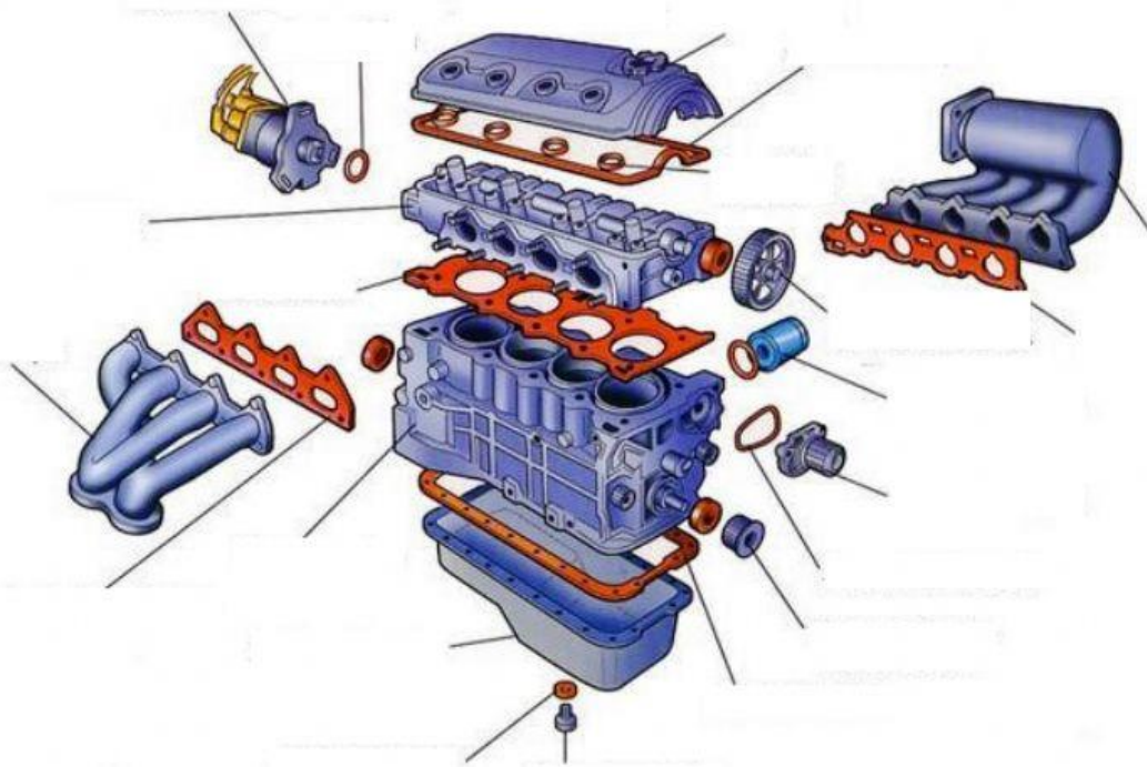
Despiece de un motor de 4 cilindros en linea
