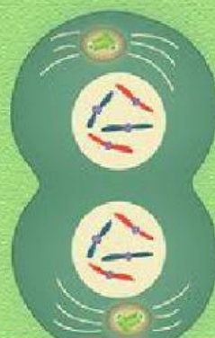
5 Telofase
