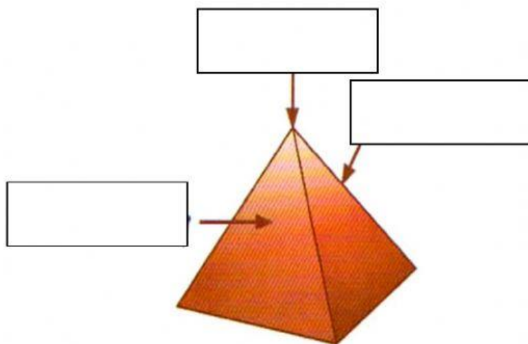
正方棱锥体
