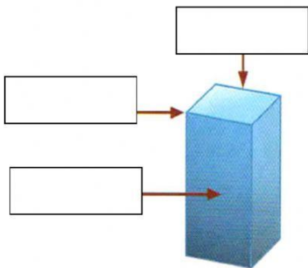
长方体
