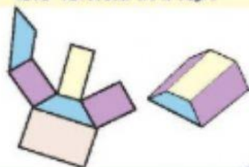
מנסרה מרובעת ופריסתה
