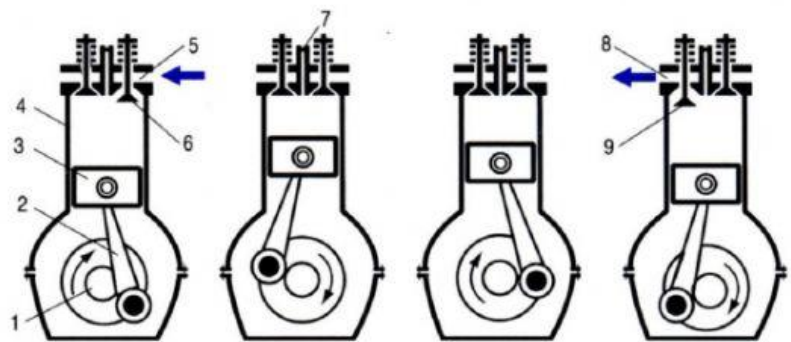
Hình 21.2: Sơ đồ chu trình làm việc của động cơ điêzen 4 kì
