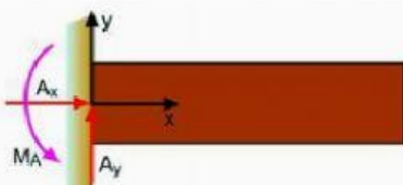
Menahan Momen, Gaya Horizontal, dan Gaya Vertikal
