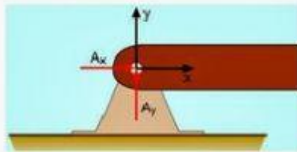
Menahan Gaya Horizontal dan Vertikal
