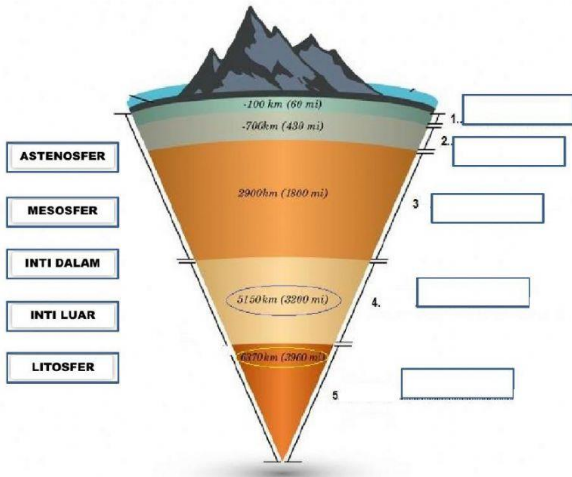
Struktur Bumi
