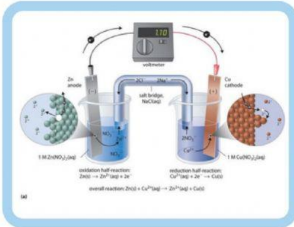
Gambar (a) Sel Volta
