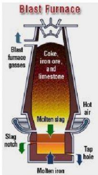
Gambar 3.3 Tanur tinggi pengolahan besi
